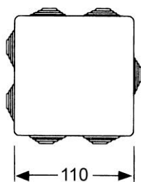
Ref. 615 7 conos para tubo de \varnothing 25 (M25).
